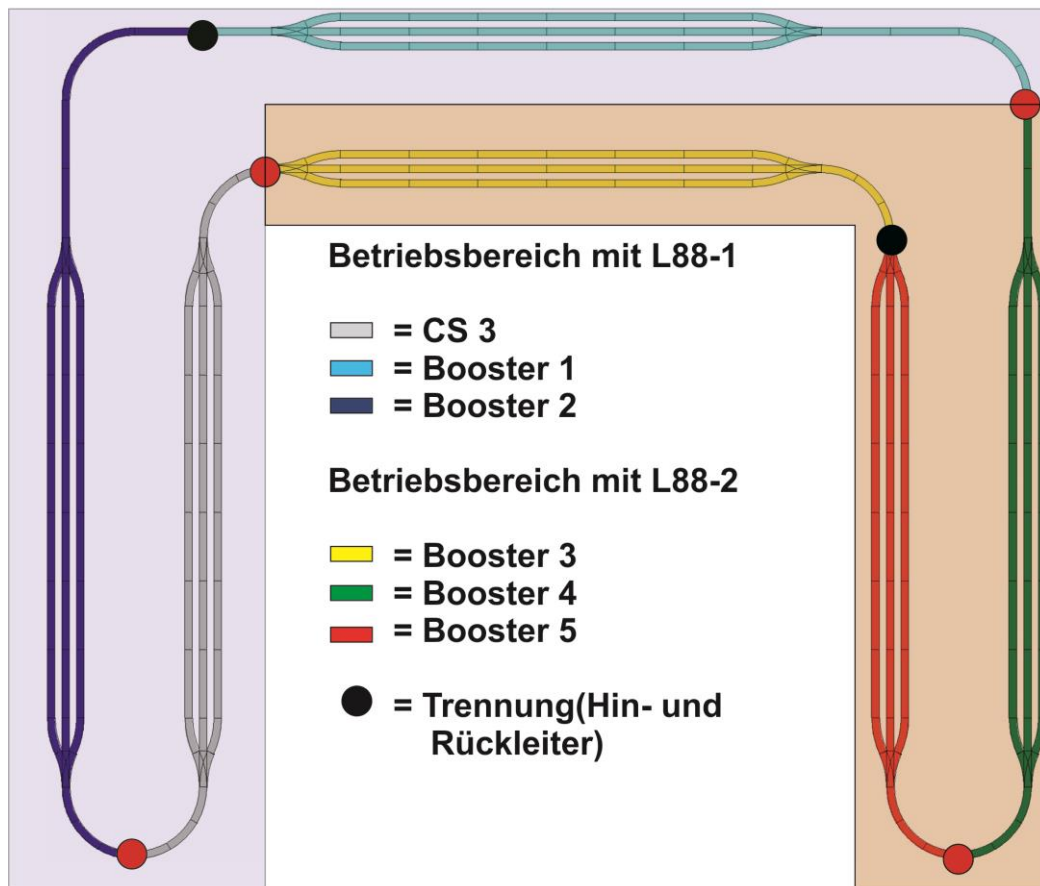
Grafik: Anlage mit 2 Betriebsbereichen
