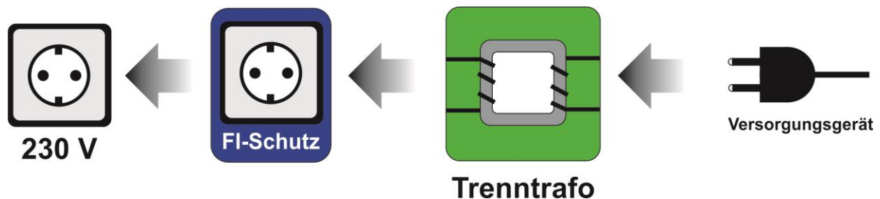
Grafik: Der zusätzliche Einsatz eines Trenntransformators erhöht die elektrische Sicherheit.
